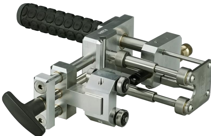
Ořezávač zoxidovaného povrchu plastových trubek 25 – 125
