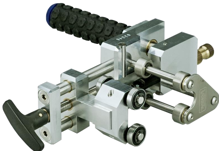
Ořezávač zoxidovaného povrchu plastových trubek 25 – 63
